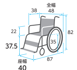
スイングアーム式 リアキャスタ
